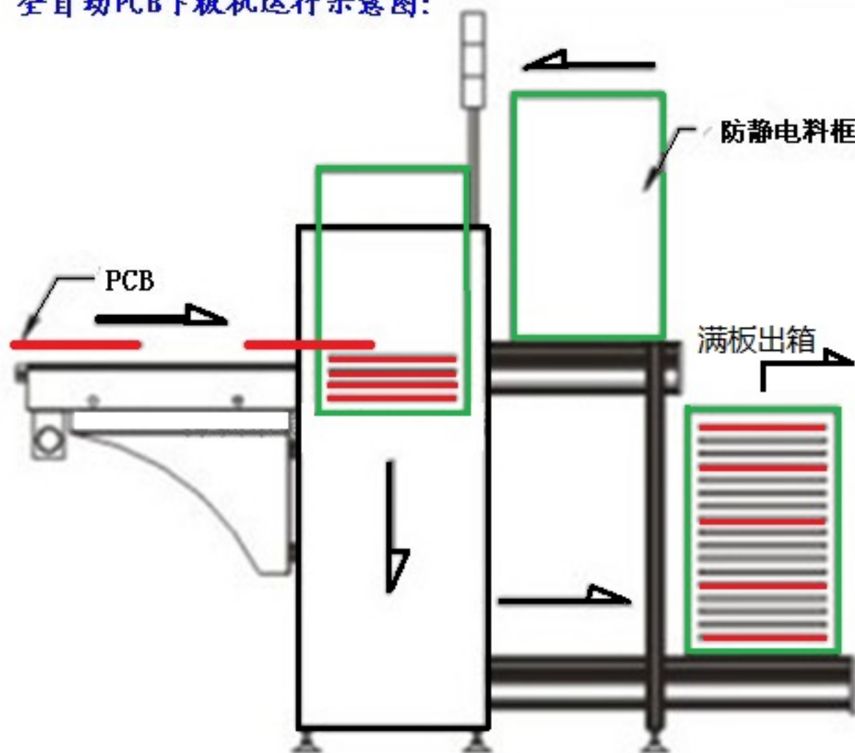
全自动PCB下板机运行示意图:
